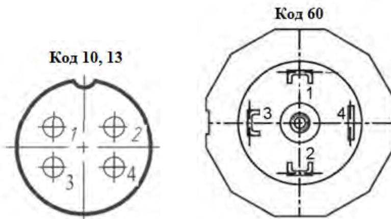
Рисунок В.1 — Схема подключения преобразователей общепромышленного исполнения с кодами 10, 13, 60 по таблице А.10
